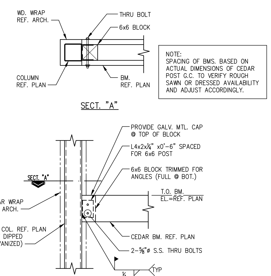
01 SECTION • TRELLIS SCALE: 3/4"=1'-0"
