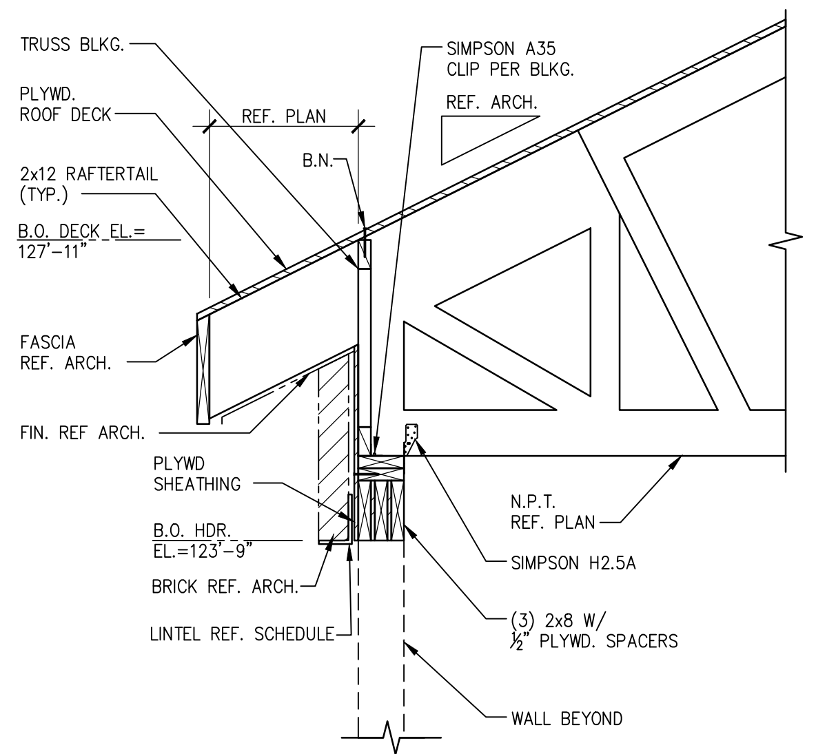
06 SECTION SCALE: 3/4"=1'-0"
