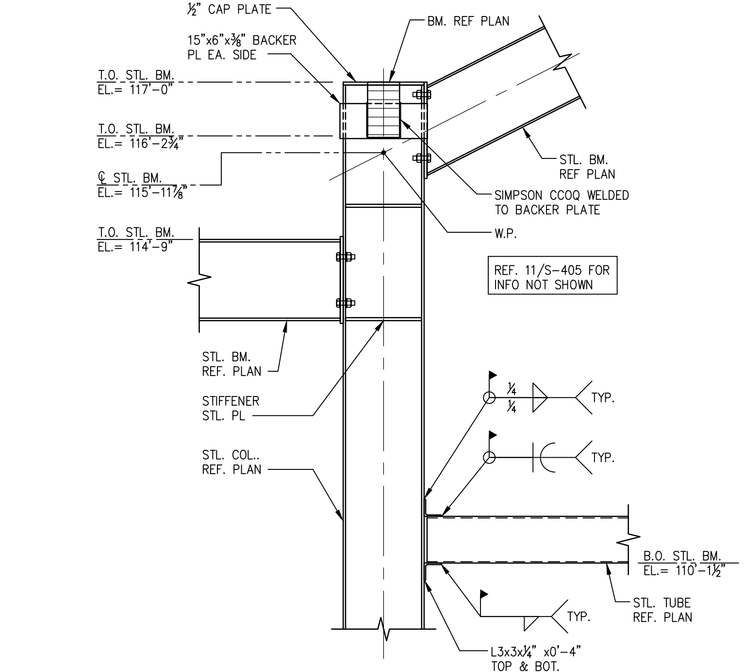
08 SECTION SCALE: 3/4"=1'-0"
