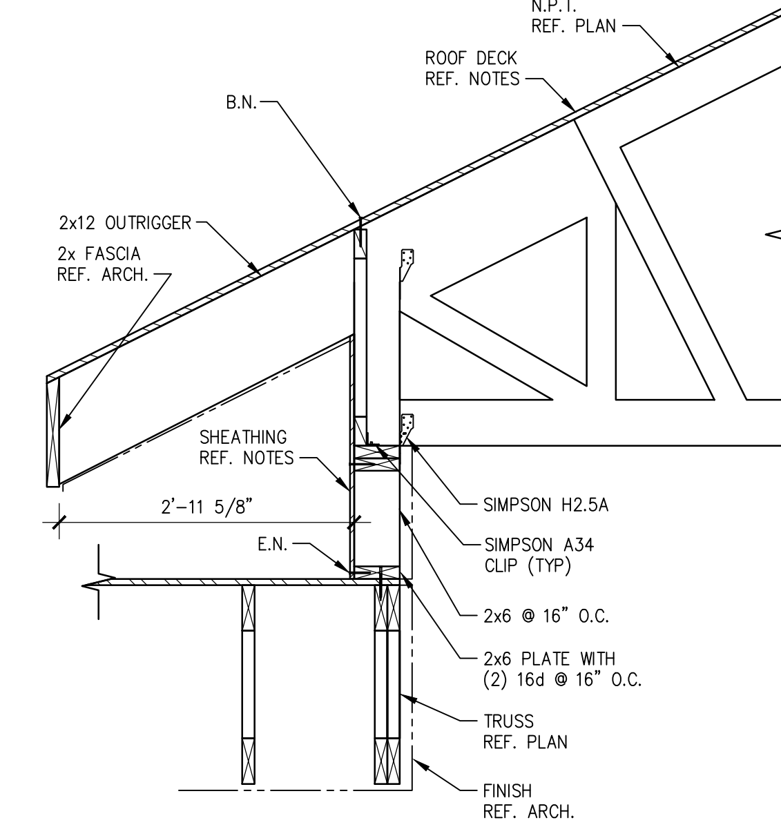
04 SECTION SCALE: 3/4"=1'-0"
