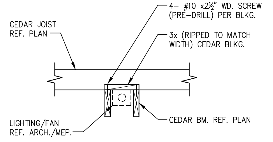
03 SECTION • TRELLIS SCALE: 3/4"=1'-0"
