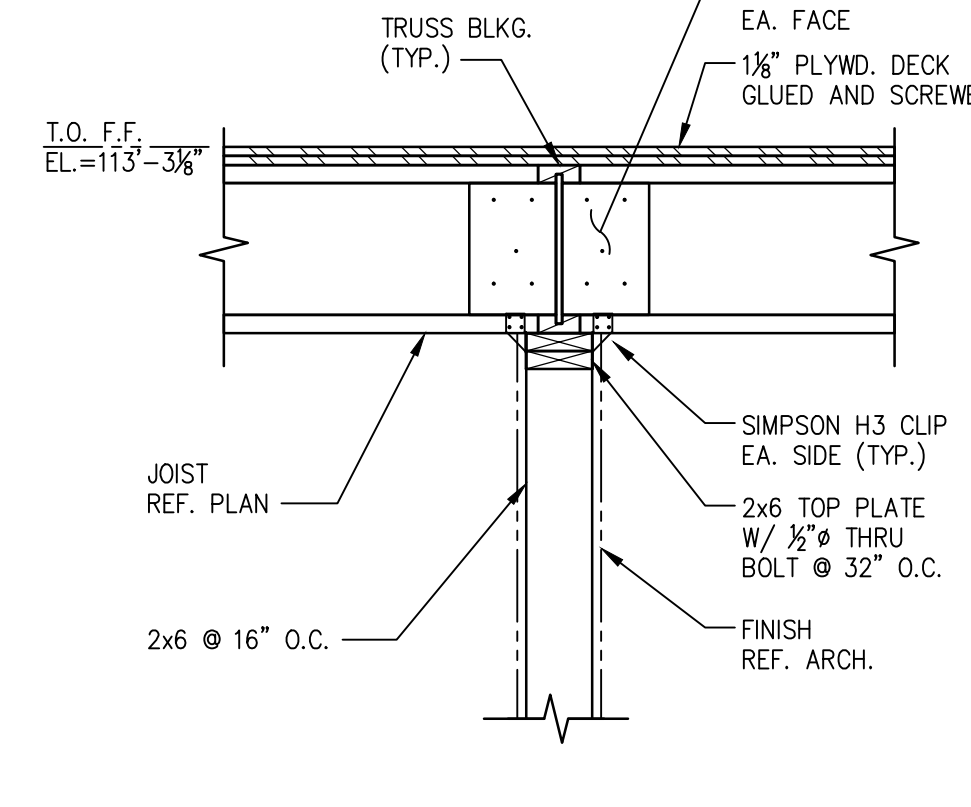
09 SECTION SCALE: 3/4"=1'-0"
