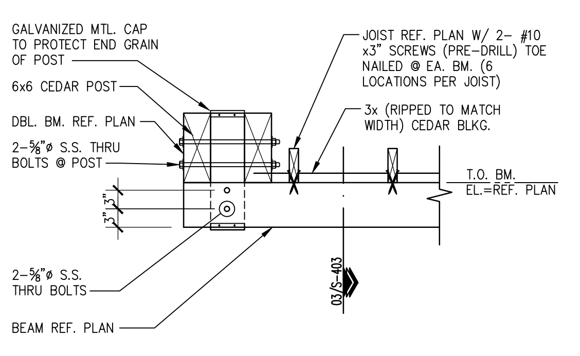
02 SECTION • TRELLIS SCALE: 3/4"=1'-0"
