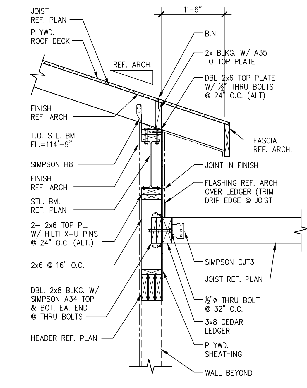
07 SECTION SCALE: 3/4"=1'-0"
