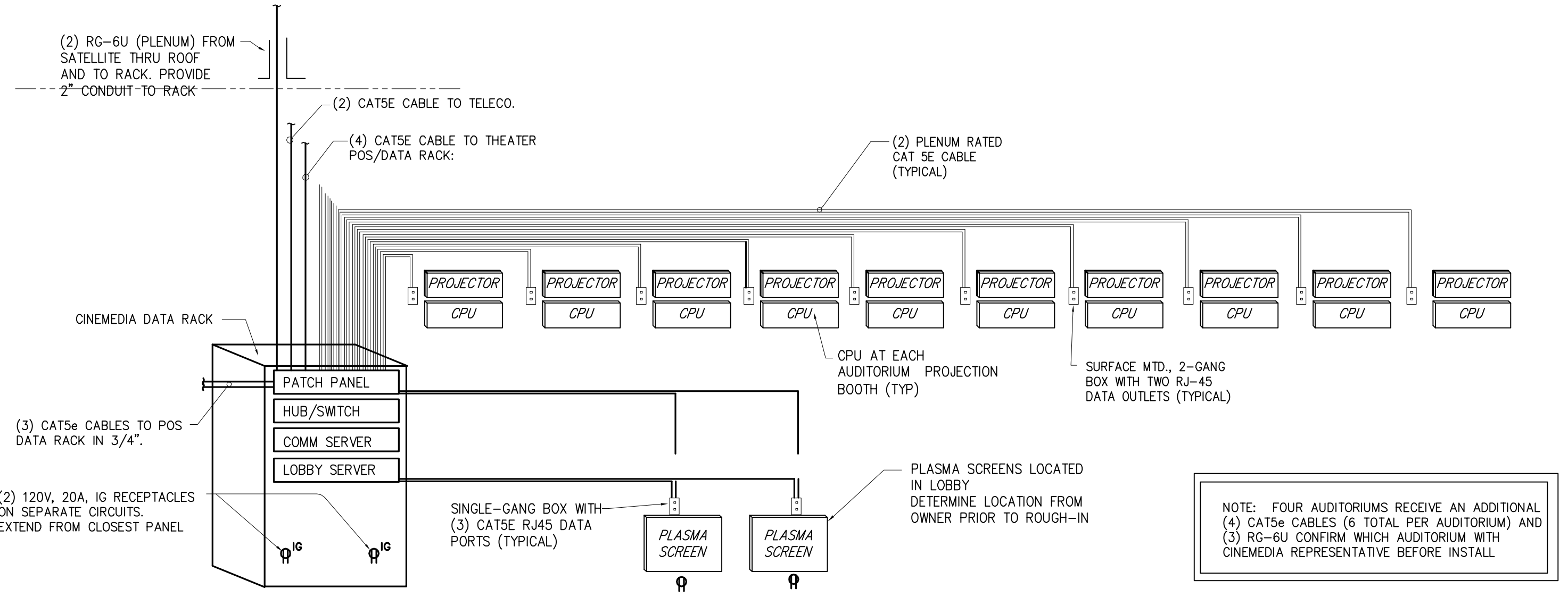
21 CINEMEDIA CAT 5E RISER DIAGRAM SCALE: NO SCALE
